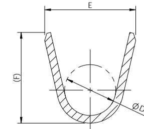
Section B-B Scale 10 : 1
